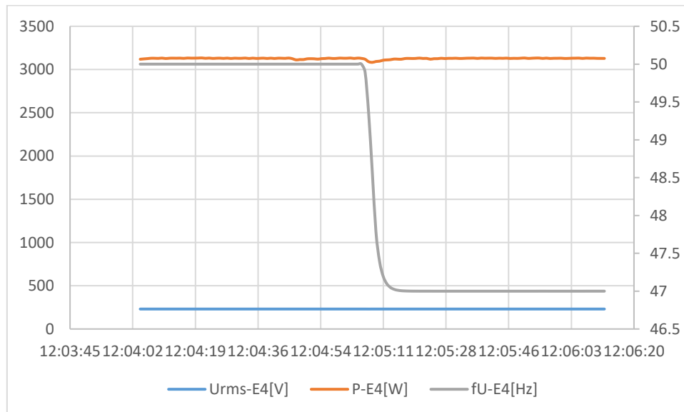
RoCoF
